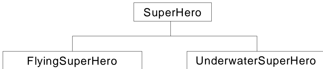
Gambar 1.1: Contoh Pewarisan
